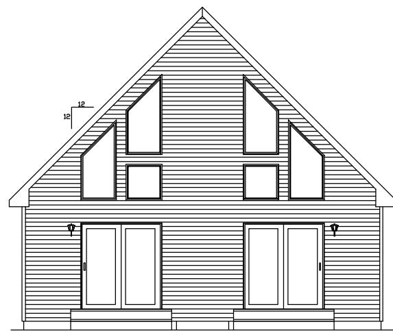
RIGHT ELEVATION
