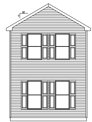
RIGHT ELEVATION
